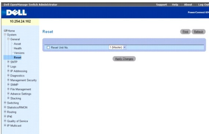
Abbildung 6-8. Zurücksetzen
