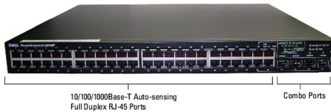
Abbildung 2-5. PowerConnect 6248P mit 48 10/100/1000-Base-T-Ports
