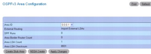
Abbildung 11-18. OSPFv3-Bereichskonfiguration - Stub Area und NSSA erstellen
